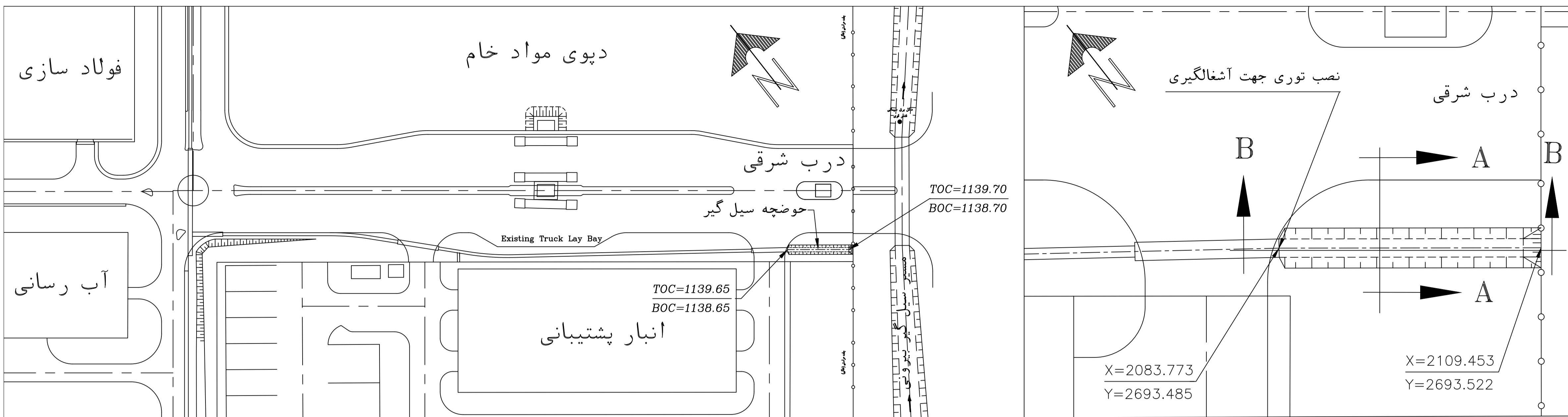
پلان موقعیت حوضچه سیل گیر SCALE 1:1
