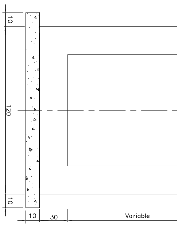
برش D-D NO SCALE FORMWORK
